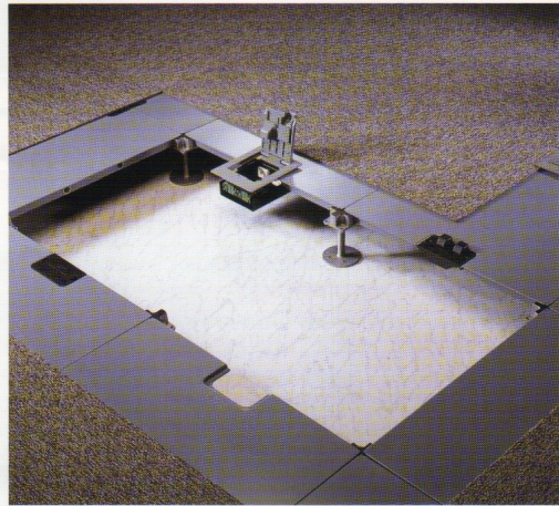
後貼式施工 (方塊地毯)
