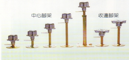
各式高度腳架 H60mm~200mm
